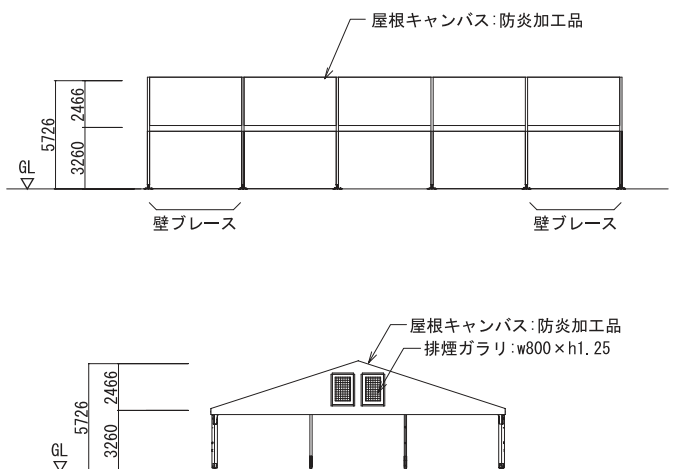
立面図
