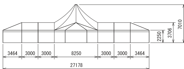
立面図
