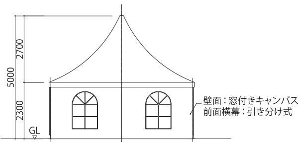
断面図
